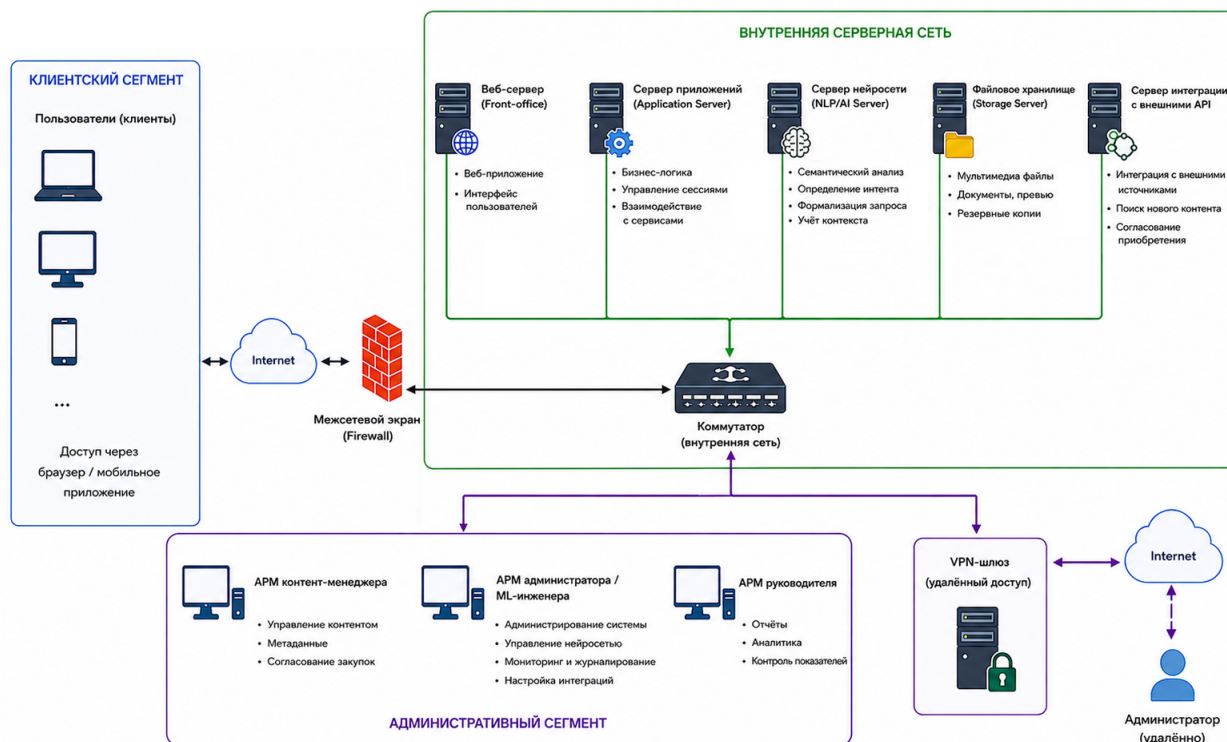
Рисунок 1 - Схема компьютерной сети
